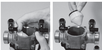
C- Fjern ventilen opstrøms (6).
