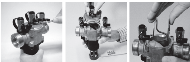
A- Fjern dækslet (3) ved at løsne skruerne (4). B- Fjern afstandsstykket (5).
