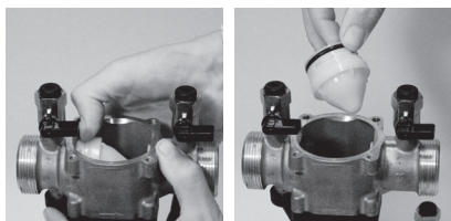
C- Rimuovere la valvola a monte (6).
