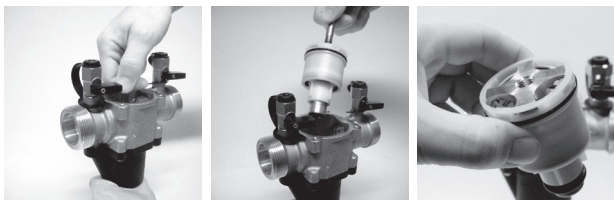
D- Rimuovere il modulo della valvola di scarico (8) con il bullone M10 in dotazione nel kit.
