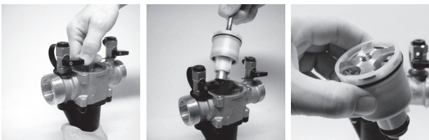
D- Fjern modulet med drænventilen (8) med møtrikken M10 der medfølger i sættet.
