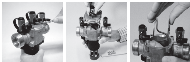
A- Rimuovere il coperchio (3) svitando le viti (4). B- Rimuovere il distanziale (5).
