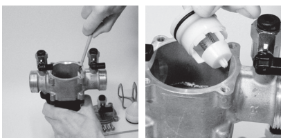
C- Fjern ventilen nedstrøms (7).
